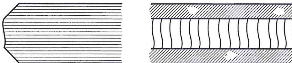
Рисунок А.1 — Притупленная кромка
